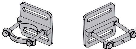
Réf. : 390100 Console de montage mural pour Mâts individuelles rondes Réf. : 390100-1 Console de montage mural pour Mâts individuelles carrées
