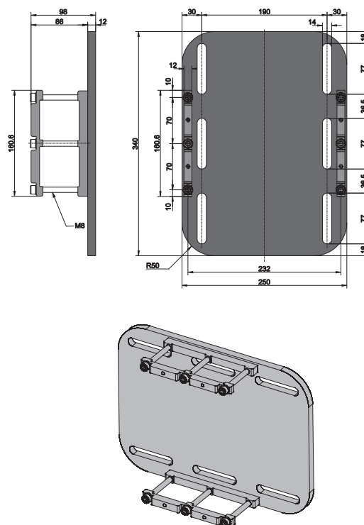
Réf. : 390402-1 Plaque de montage à pince pour Mâts doubles carrées
