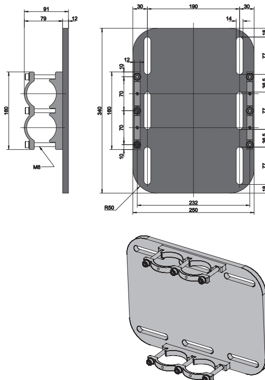
Réf. : 390402 Plaque de montage à pince pour Mâts doubles rondes
