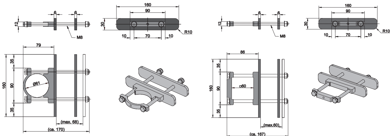
Réf. : 390356 Console de montage de garde-corps pour Mâttes individuelles rondes
