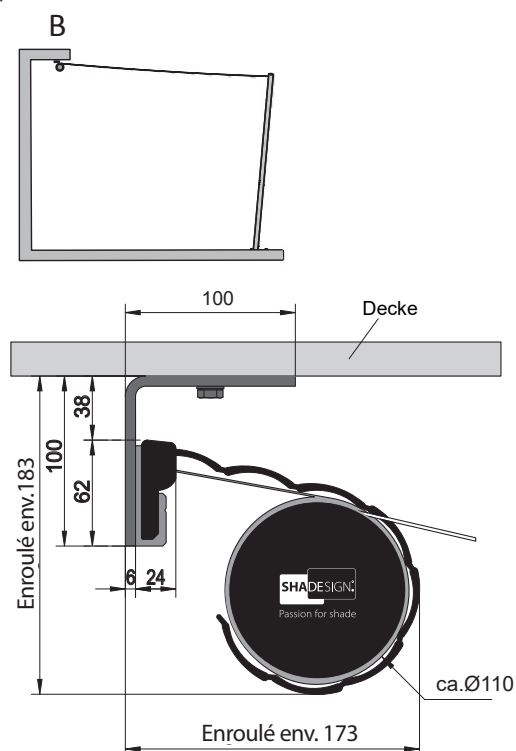
Vue détaillée B : Montage au plafond (avec toit de protection)
