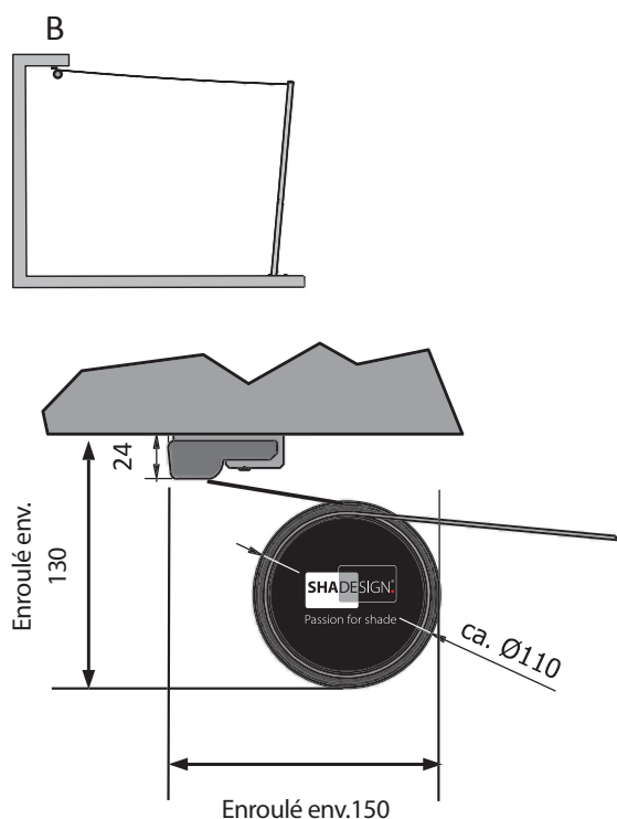
Vue détaillée B : Montage au plafond (sans toit de protection)
