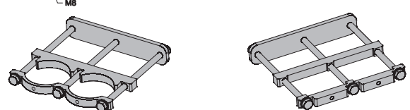
Réf. : 390503 Console de montage avec contre-dalle pour doubles Mâts rondes Réf. : 390503-1 Console de montage avec contre-dalle pour doubles Mâts carrées
