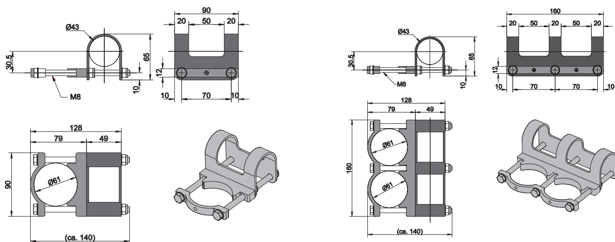
Réf. : 390160 Console de montage de garde-corps pour Mâttes individuelles rondes
