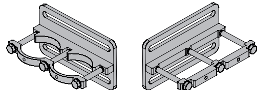
Réf. : 390501 Console de montage mural pour double Mât ronde Réf. : 390501-1 Console de montage mural pour double Mât carrée
