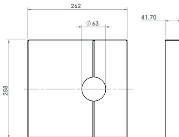
Couverture de dalle de sol en 2 parties, enfichable
