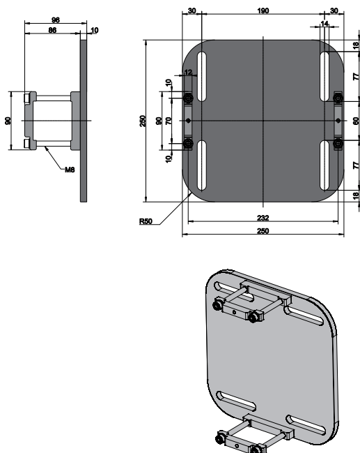
Réf. : 390401-1 Plaque de montage à pince pour Mâts individuelles carrées
